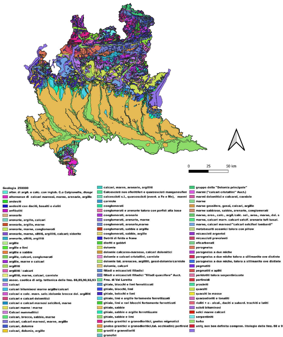
Fig. 3 – Mappa litologica della Lombardia ( https://www.geoportale.regione.lombardia.it/ )
